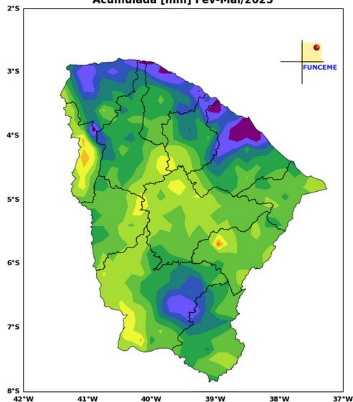
Precipitação Acumulada [mm] Fev-Mai/2025
