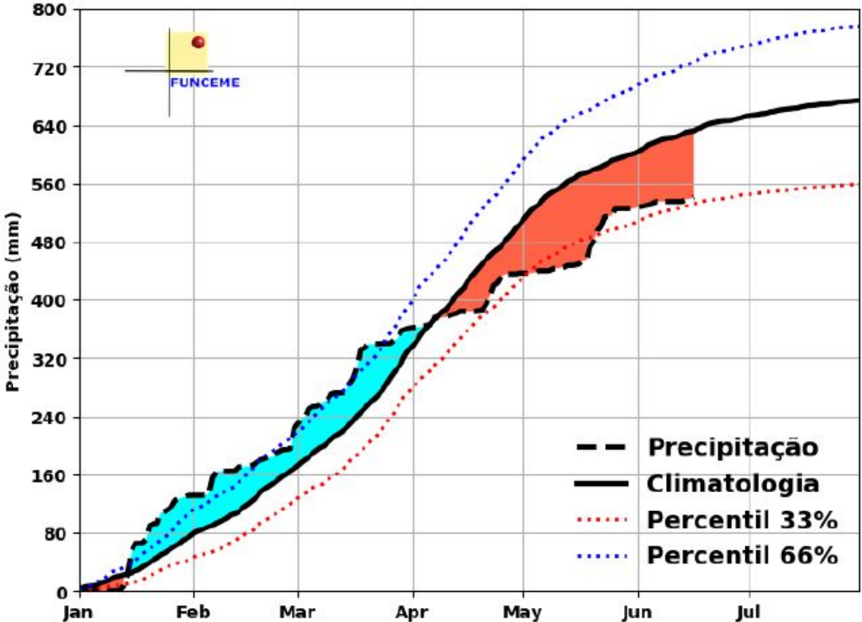
Banabuiú Precipitação acumulada de 01/Jan - 16/Jun/2025
